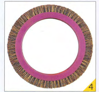
德国毛刷轮 φ 180 × φ 123 × 21.5
