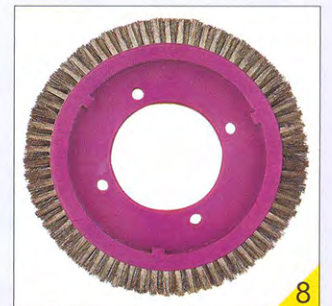
乘福机毛刷轮 (Chengfn) φ 182 × φ 72 × 22
