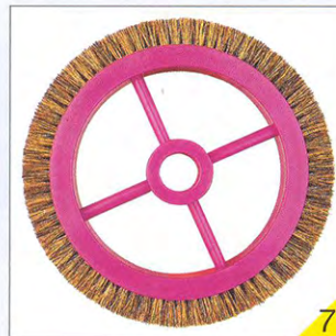
立信门富士小毛刷轮 (Monforts) φ 182 × φ 23 × 26
