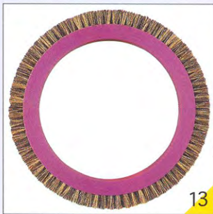
阿托斯毛刷轮 (Artos) φ 205 × φ 145 × 17
